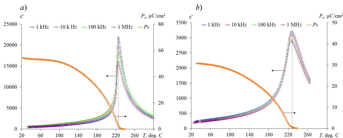
Рис. 4. Температурные зависимости диэлектрической проницаемости и спонтанной поляризации для образцов плотной (а) и пористой (b) керамик (\text{Pb}_{0.9}\text{Ba}_{0.1})(\text{Zr}_{0.9}\text{Ti}_{0.1})\text{O}_3 .
