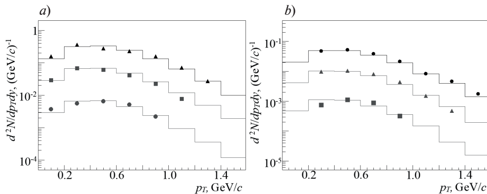
Рис. 4. Исходные (линии) и восстановленные (символы) спектры рождения K^*(892)^0 - (a) и \phi(1020) - (b) резонансов для столкновений Xe + W при энергии E_{kin} = 2,54 ГэВ в области быстрот -1,0 < y_{CMS} < 0,0 . Рассмотрены 3 диапазона по центральности, %: 0 – 20 (▲), 20 – 40 (■) и 40 – 90 (•).
